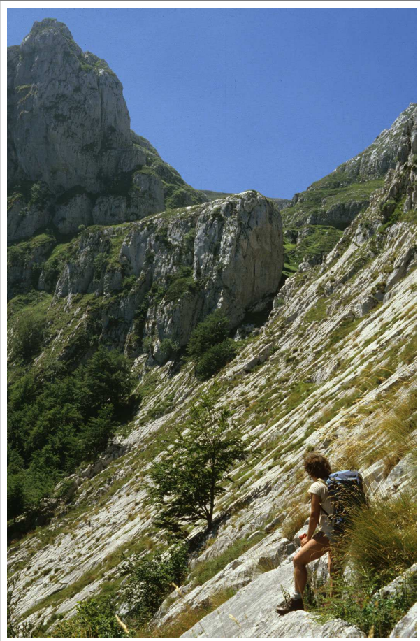
L'entrée de la cueva de Castেলাgua (n°415) s'ouvre au pied de l'unique arbre de ce lapiaz incliné. La pente n'est pas liée au pendage général des couches mais à la présence d'une lentille récifale (capping-beds).
