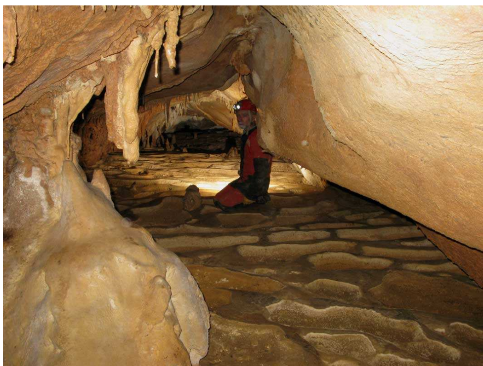
Les gours dans la galerie d'entrée de la cueva 405.
