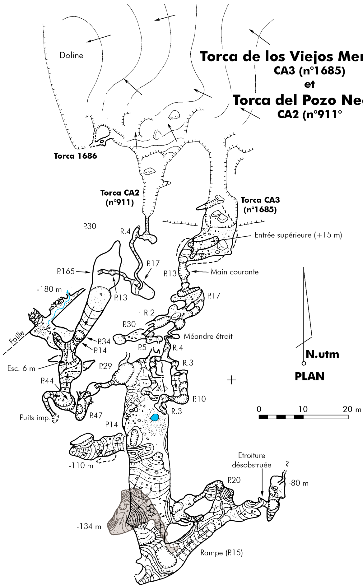
Topographie Pozo Negro (n°911) : SGCAF 1982 (Ph. Morverand) Torca de los Viejos Mendrugos (n° 1685) : S.C.Dijon 2012-2013 (G. Aranzabal, J. Argos, D. Boibessot, E. Bunoz, P. et S. Degouve, I. Expósito, Ch. Philippe, B. Pernot, G. Simonnot)
